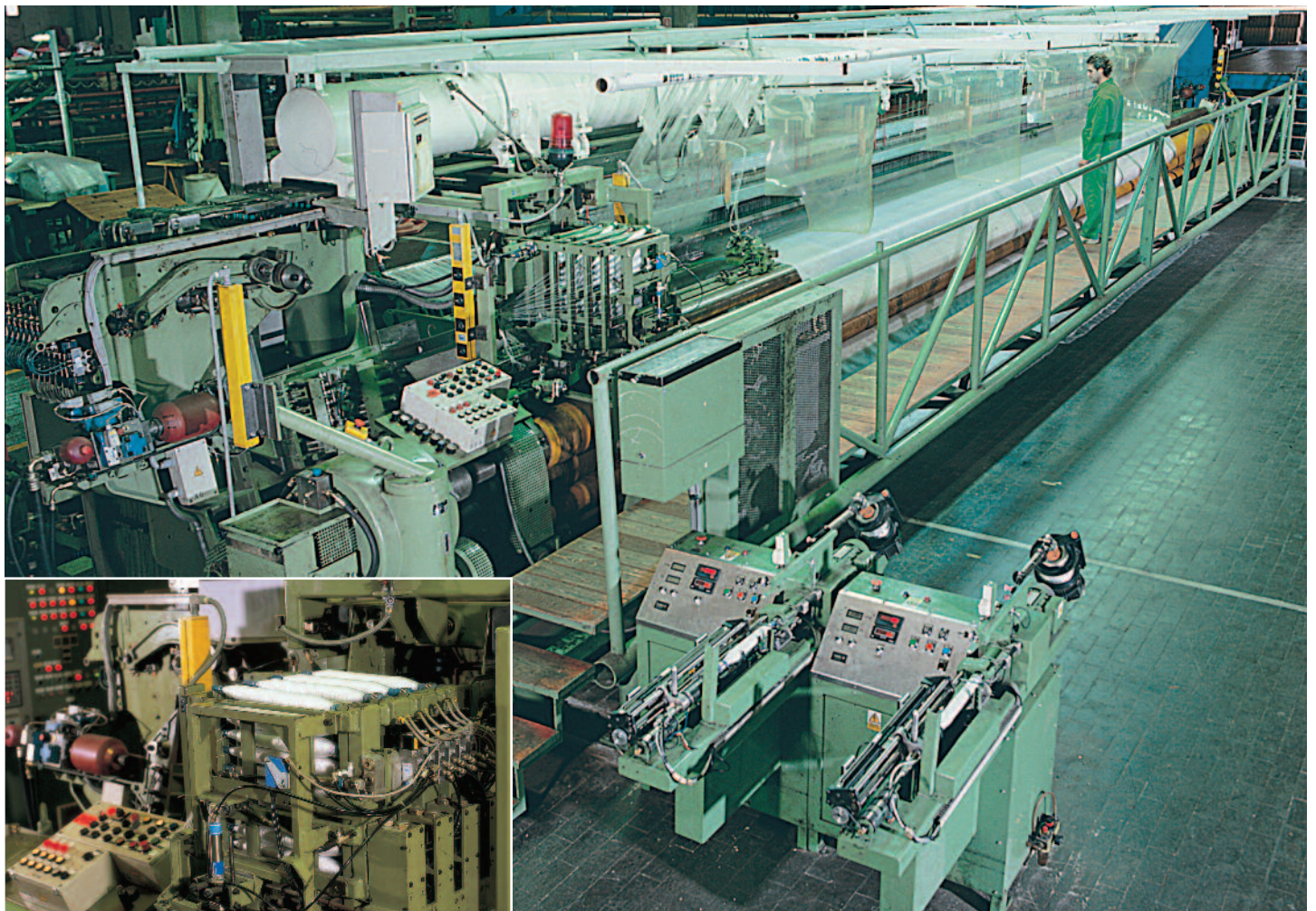
Telaio automatico da mt. 14,00 per tessuti di base per feltri umidi
