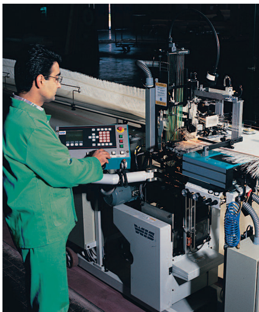
Macchina automatica per giunzioni di tele essiccatrici
