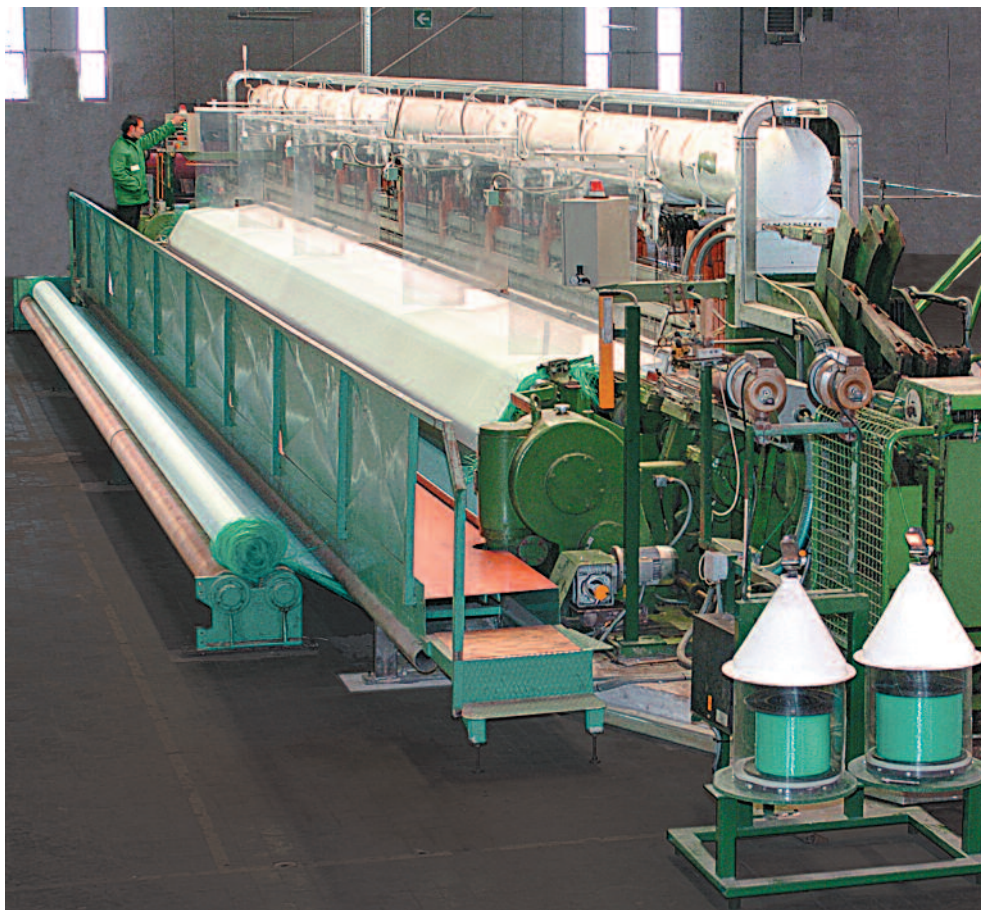
Telaio a pinze da mt. 14,50 per tele di seccheria
