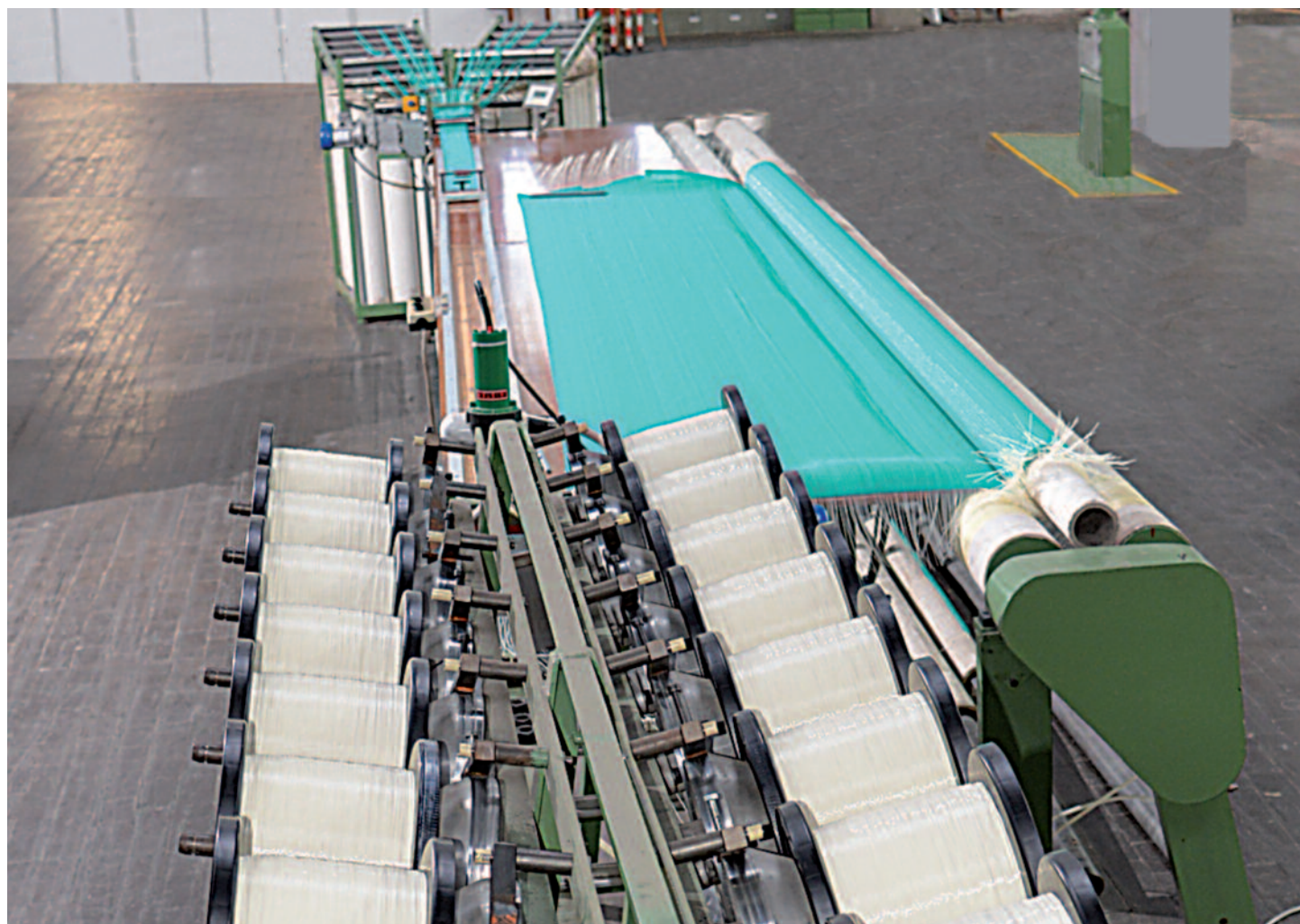
Assemblatrice tele multispirali
