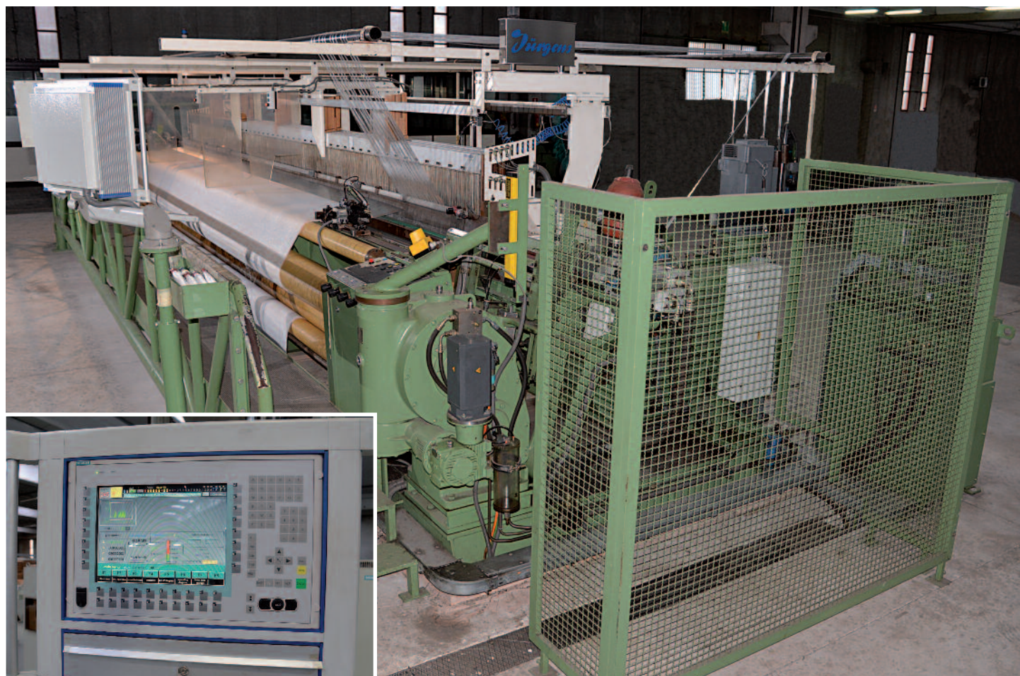
Telaio da mt. 8,50 per tessuti di base per feltri umidi
